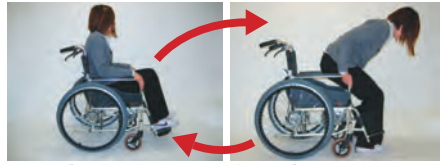
自動ブレーキ装置 “歯”でブレーキを掛けるため 高い静止力で車いすを止め られます。
